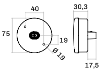
Fixação frontal
