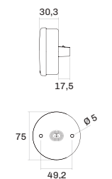
Fixação traseira
