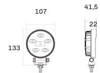
2340 - 5RD - Redondo
