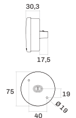
Fixação frontal
