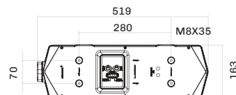
Fixação traseira
